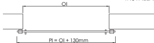
PORTA SINGOLA E PORTA A DUE ANTE CONTRAPPOSTO PER INSTALLAZIONE SU PARETE
